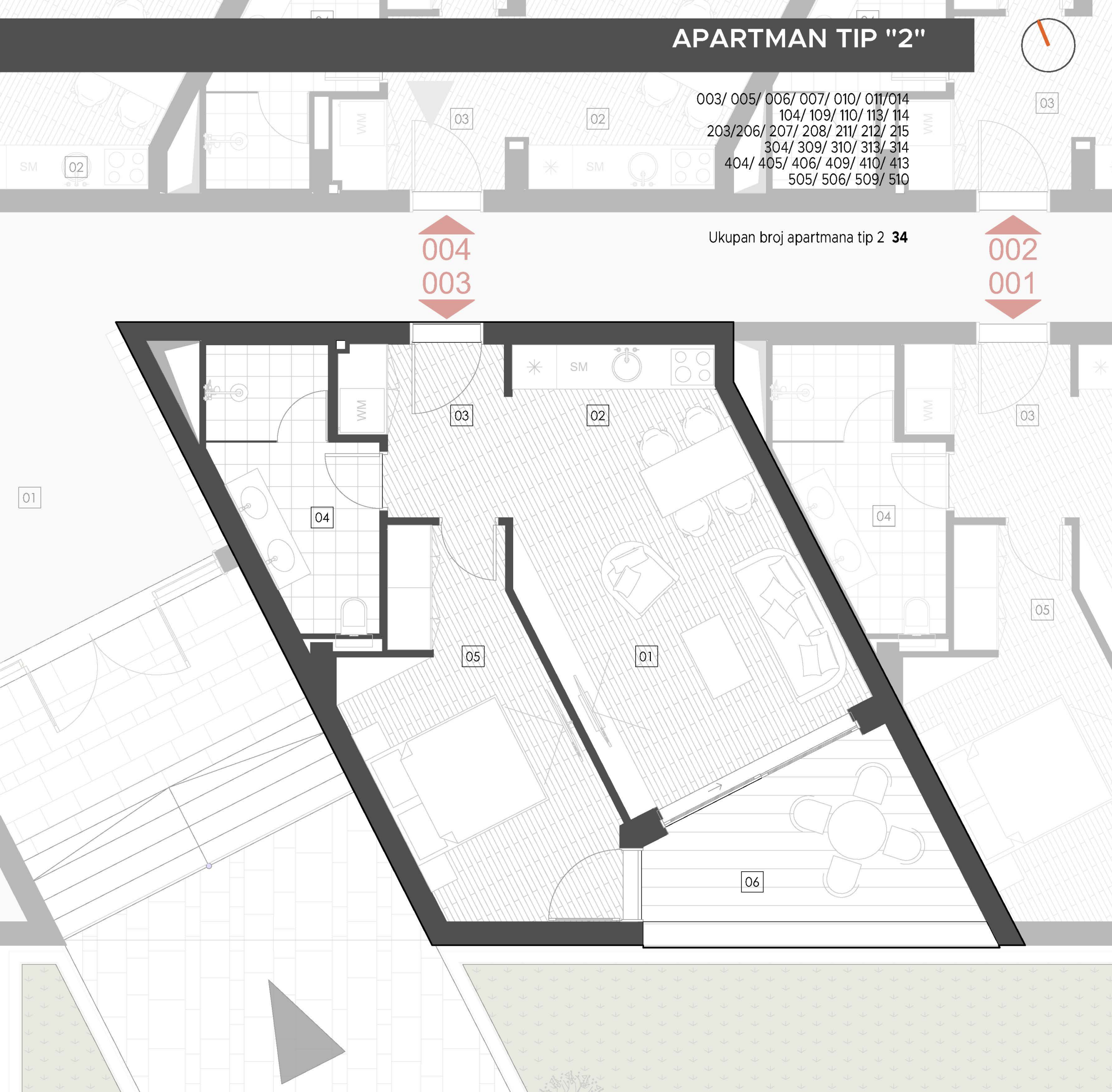
Osnova Prizemlja
